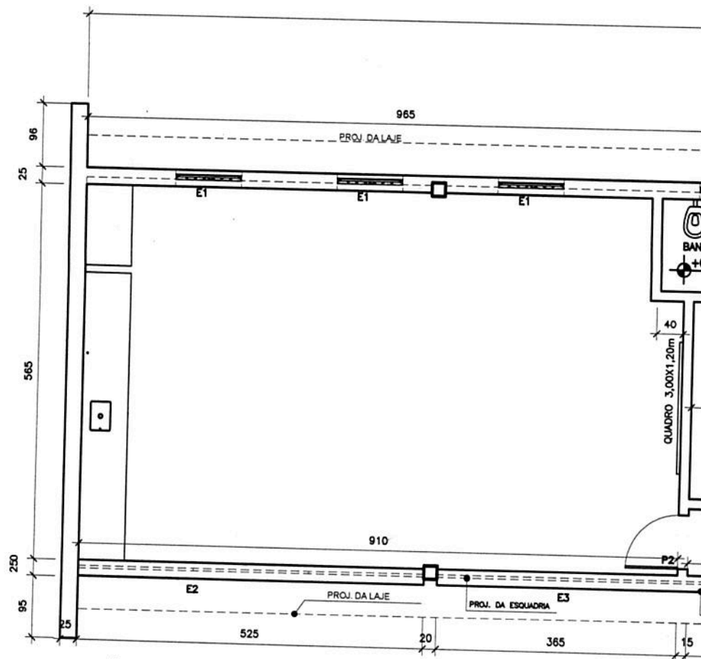
2 PLANTA BAIXA 1º PAVIMENTO ESCALA ----- 1:75
